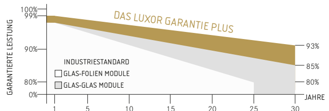
Lineare Leistungsgarantie 1
