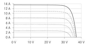
UI-Kennlinie Bsp. LX-400M / 182-108+
