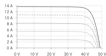
UI-diagram e.g. 540Wp
