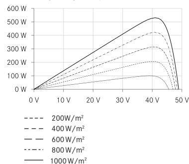
UP-diagram e.g. 540Wp
