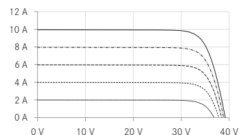
UI-diagram e.g. LX-310M/158-60+
