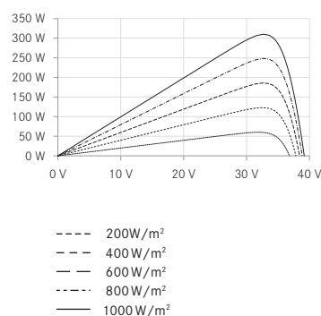
UP-diagram e.g. LX-310M/158-60+
