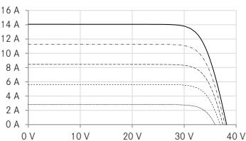
UI-Kennlinie Bsp. 420 Wp
