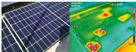
Abb. 2 Verschattung und Hotspots durch Blitzfangstange 2
