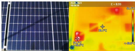
Abb. 1 Verschattung und Hotspots durch Blitzfangstange 1
